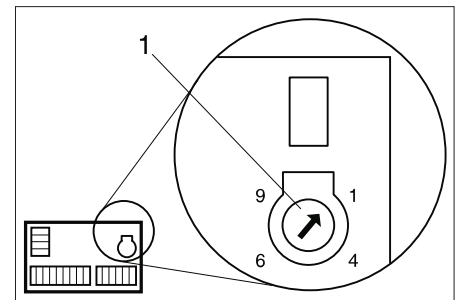
1 Drehpotentiometer
