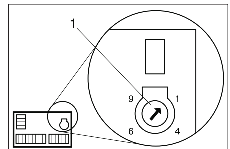
1 Sukamasis potenciomėtras
