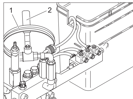
1 Utluftingsslange
