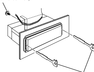
Принадлежность ② Приспособление для снятия
