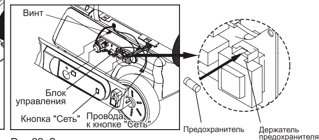
Рис 22. Замена предохранителя
