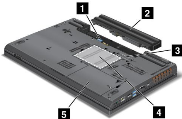
Рис. 4. ThinkPad T530, T530i и W530 (вид снизу)
