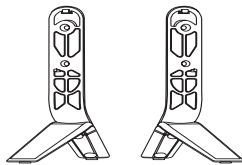
Suport Assy (Corpul suportului / Baza suportului) (Doar 70LB65**-ZA, LB67**, LB68**, LB69**, LB72**, LB73**-ZA) (Consultați p. A-3)
