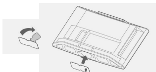
Захисна кришка
