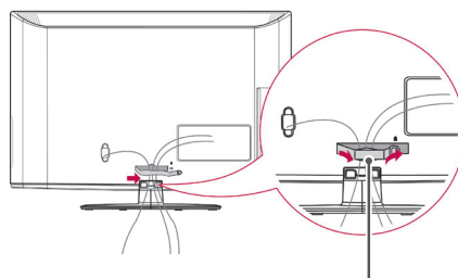
Хомут для фиксации проводов
