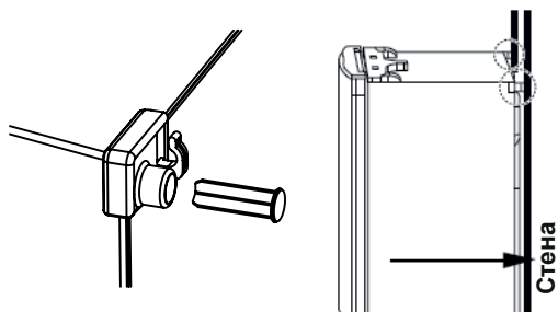
Рис. 2. Установка ограничительных упоров
