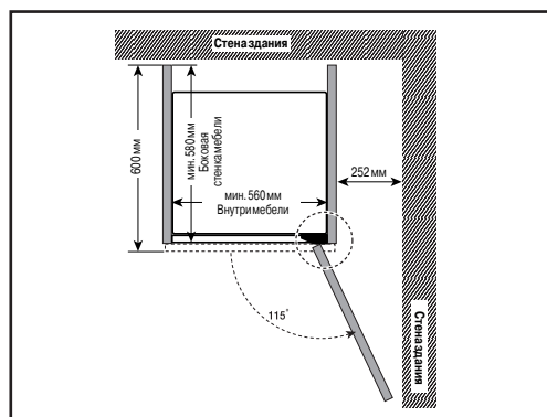
■ Примерный план-чертеж установочного шкафа и максимального раствора двери
