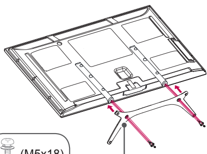
Основание подставки
