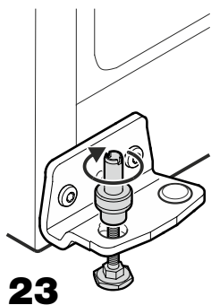
23. Вставьте ножку снизу и закрутите штифт.
