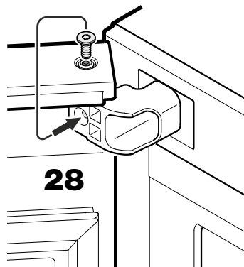
28. Выкрутите винт из опорного штифта и закрутите в отверстие шарнирного уголка.
