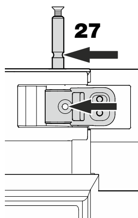
27. Вставьте опорный штифт таким образом, чтобы паз штифта оказался на одной линии с отверстием шарнирного уголка.
