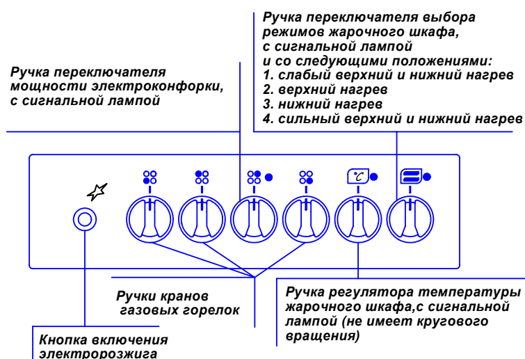
Рис. 4. Передняя панель плиты ЭГ1/3г01-2п; ЭГ1/3г01-2с
