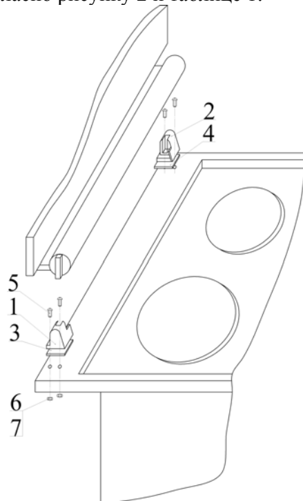
Рис. 2 Установка стеклянной крышки стола.
