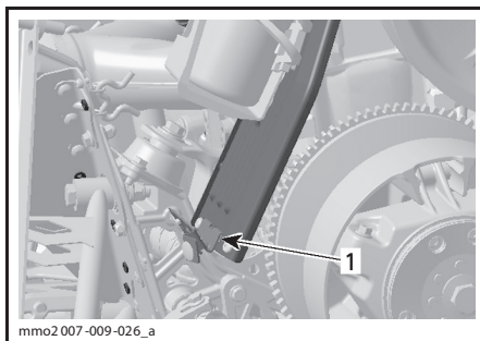
1. Пазы
