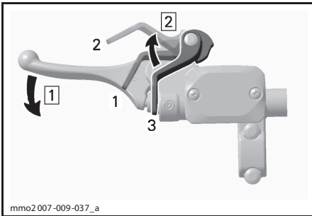
ТИПОВОЙ ВАРИАНТ — ВКЛЮЧЕНИЕ СТОЯНОЧНОГО ТОРМОЗА.
