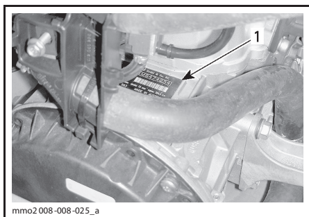
ДВИГАТЕЛЬ 600 НО Е-ТЕС® — ПРАВAYA СТОРО- НА МОТОРНОГО ОТСЕКА 1. Номер двигателя
