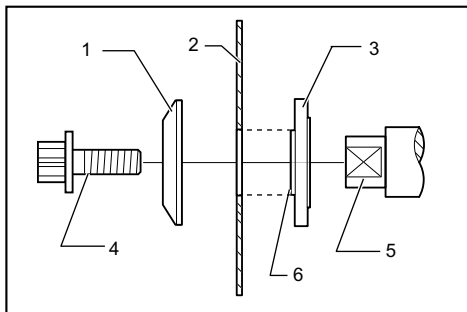
► 1. Наружный фланец 2. Пильный диск 3. Внутренний фланец 4. Болт с внутренним шестигранником (с левой резьбой) 5. Шпиндель 6. Компонент для установки диска
