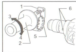
1. Основа рукоятки 2. Боковая ручка 3. Ослабить 4. Затянуть 5. Зубья 6. Выступ
