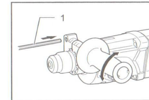
1. Глубиномер
