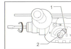
1. Кнопка блокировки 2. Ручка изменения режима работы
