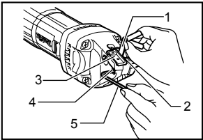
1. Calibrador de grosor 2. Superficie de cuchilla central 3. Cuchilla lateral 4. Perno hexagonal de la cabeza de conexión 5. Llave hexagonal
