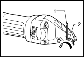
1. Llave hexagonal 2. Tornillo
