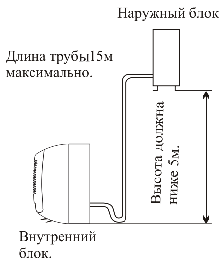
Монтажная схема
