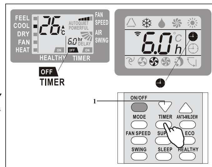
Комнатный дисплей
