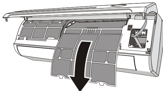
Регулировать фильтр
