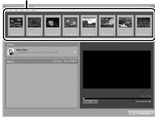
Панель «Компоненты»
