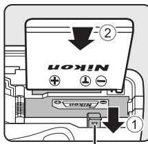
Защелка батареи
