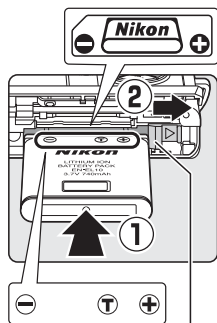
Защелка батареи
