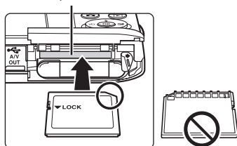
Гнездо карты памяти
