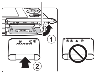
Защелка батареи
