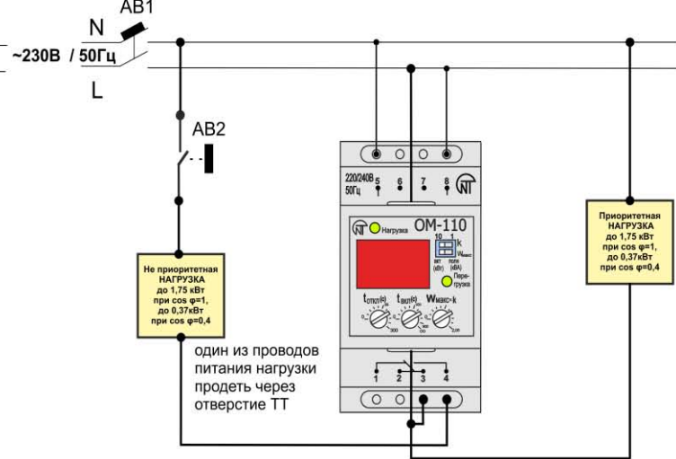
Рисунок 2 – Схема подключения OM-110
