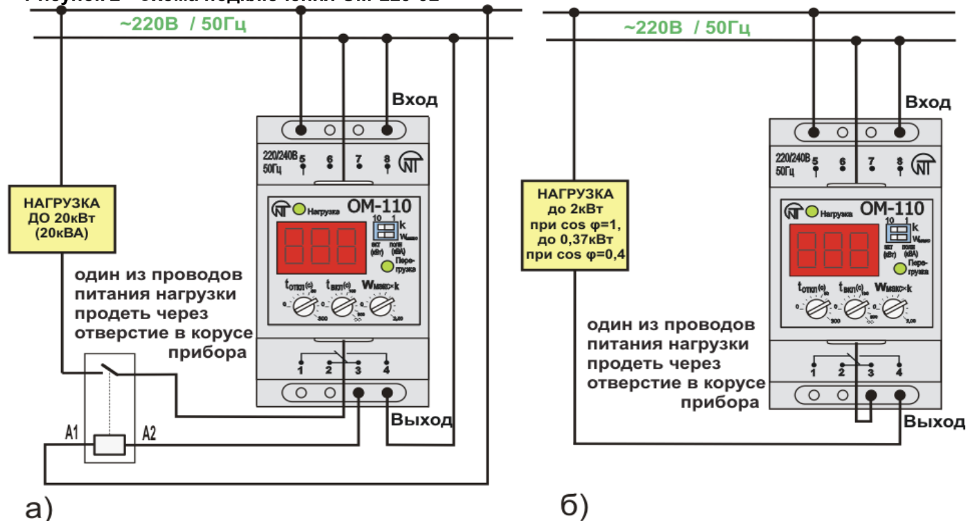
Рисунок 2 - Схема подключения ОМ-110-01
