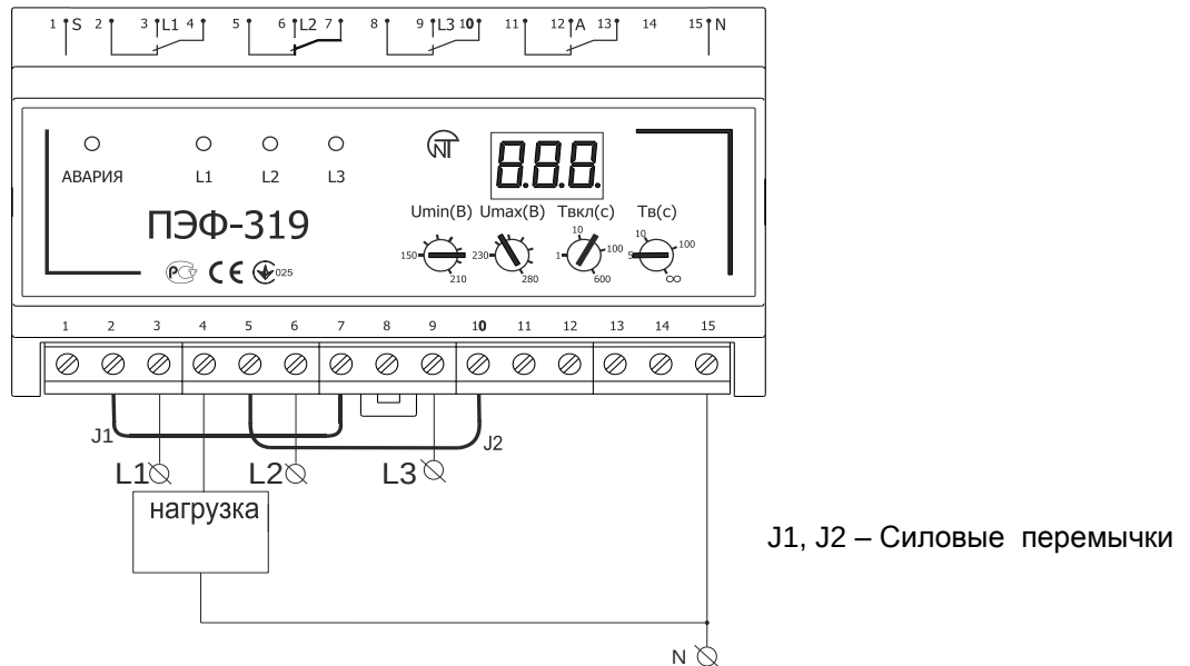
Рисунок 2 – Схема подключения ПЭФ-319 при величине нагрузки до 30 А
