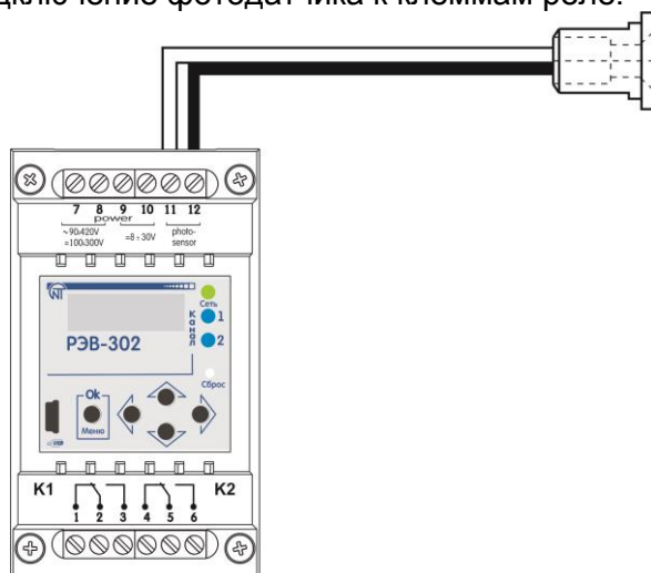
Рисунок 1.3 - Подключение фотодатчика к РЭВ-302
