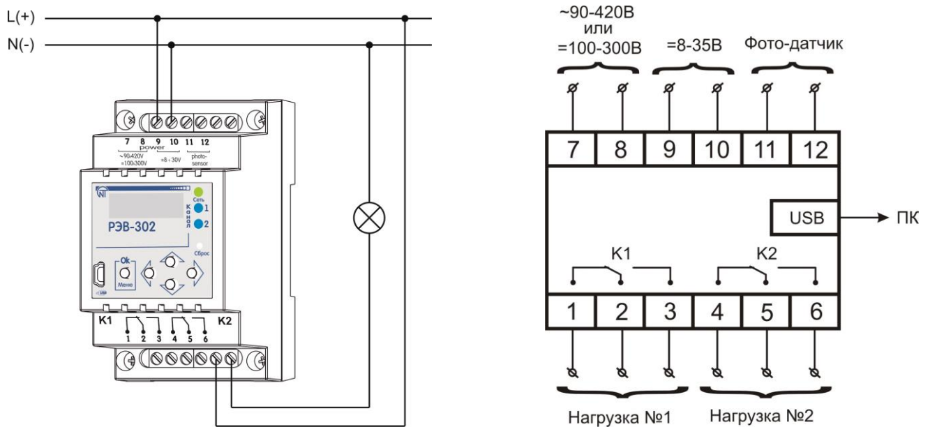
Рисунок 2.1 - Электрические соединения РЭВ-302
