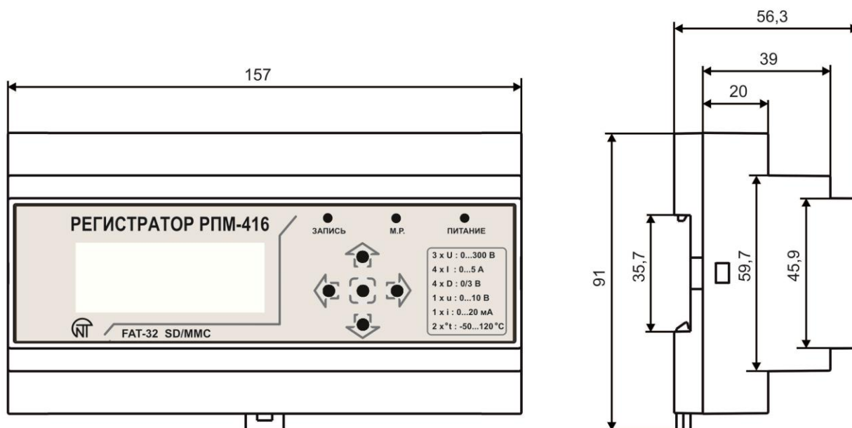
Рисунок 1.1 – Внешний вид и габаритные размеры регистратора
