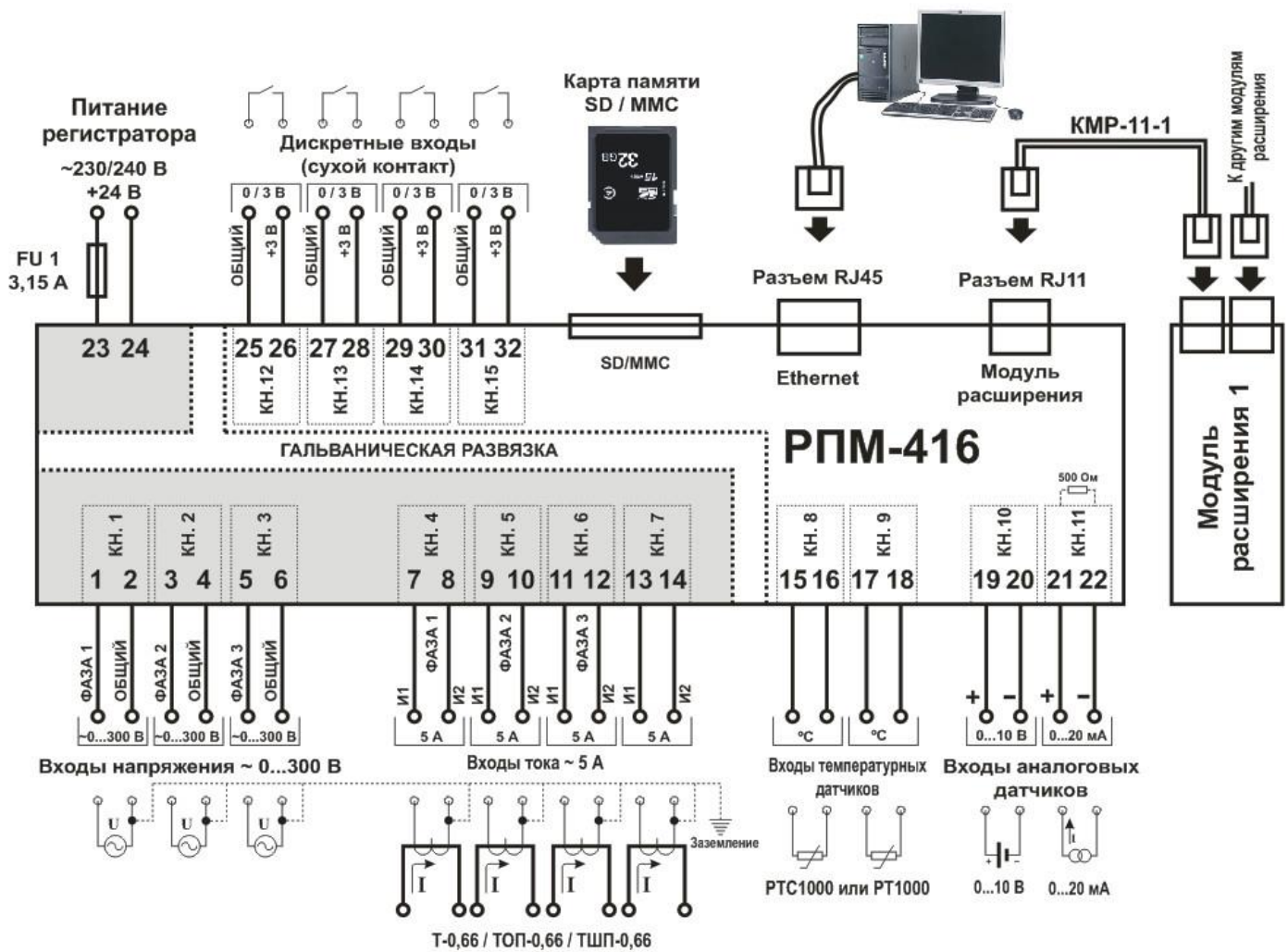
Рисунок 5.1 – Схема подключения РПМ-416
