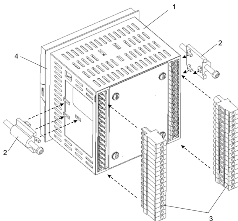
Рисунок 5.1 – Монтаж изделия
