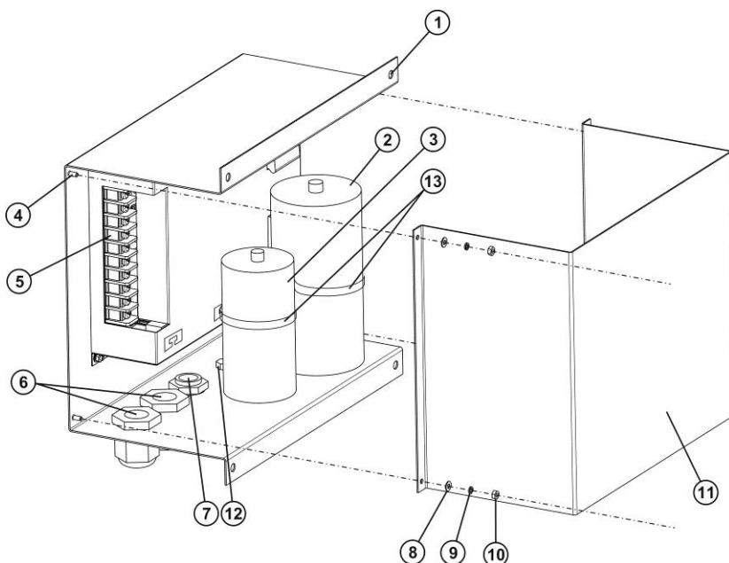
Рисунок 9 – Схема монтажа прибора
