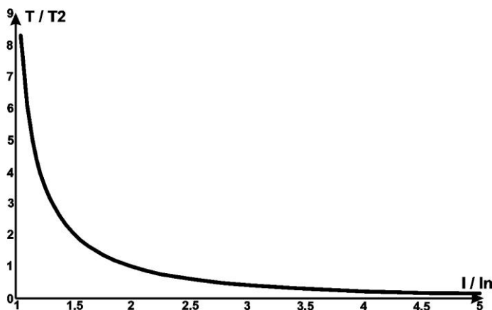
Рисунок 7 – Токо-временная характеристика
