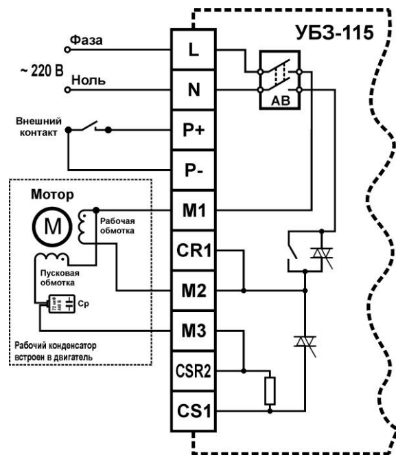
В – двигатель со встроенным рабочим конденсатором
