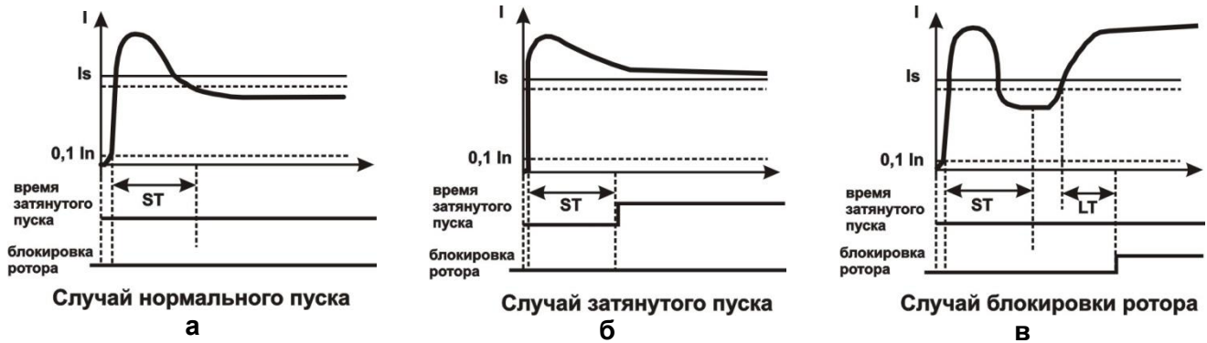
Рисунок 5 – Затынутый пуск и блокировка ротора
