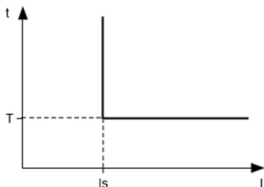
Рисунок 3.1 – Принцип защиты с независимой выдержкой времени
