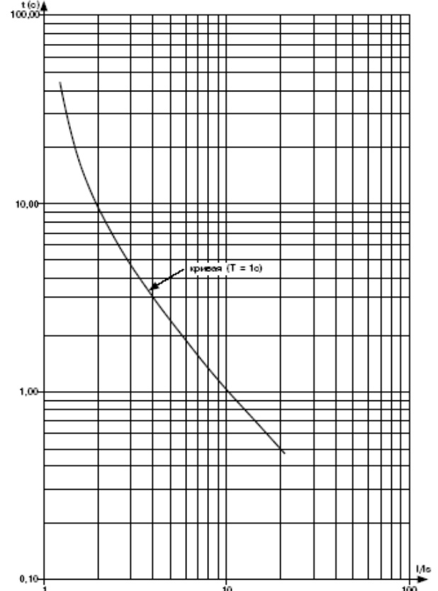
Кривая очень обратно зависимой выдержки времени VIT или длительно обратно зависимой выдержки времени LTI
