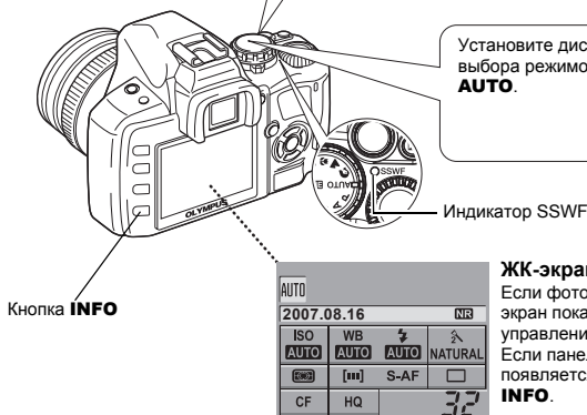
Окно панели управления
