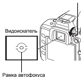
Шкала настройки диоптрий
