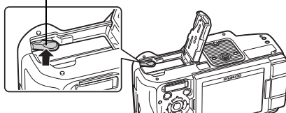
Защелка аккумулятора
