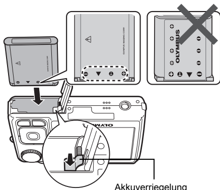
Akkuverriegelung
