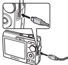
Универсальный разъем Крышка разъема
