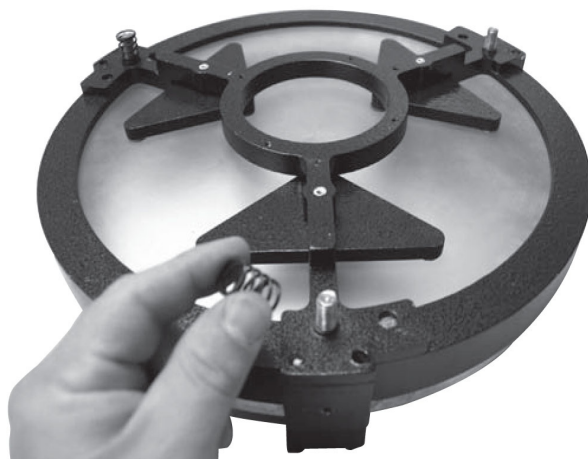
Рисунок 3. Наденьте пружины на три стержня с резьбой на корпусе зеркала.
