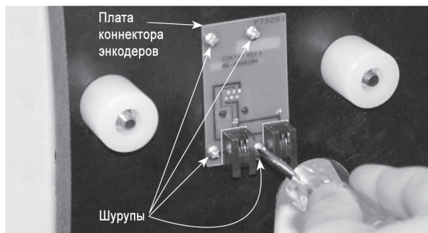
Рисунок 13. Монтаж платы коннектора энкодеров.
