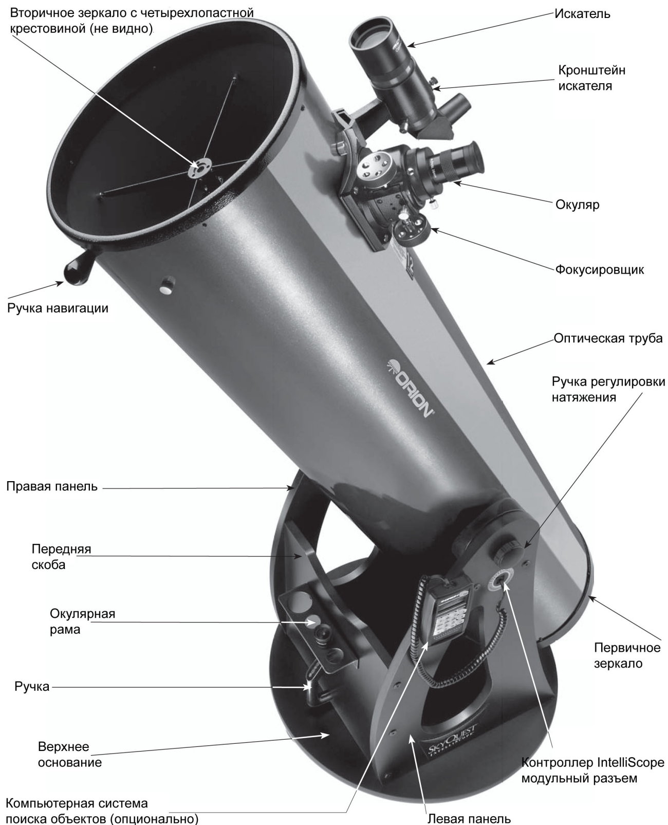
Рисунок 1. Телескоп SkyQuest XT12 IntelliScope
