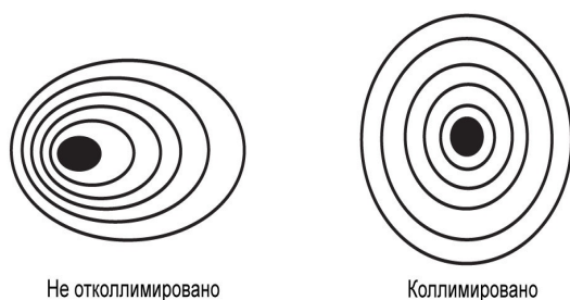
Рисунок 28. Тест по звездам покажет Вам, правильно ли отколлимирована оптика. Если оптика отколлимирована правильно, то в окуляре Вы увидите несфокусированный вид яркой звезды, как показано на правом рисунке. Если же круги не симметричны, как показано слева, значит телескопу необходима коллимация.
