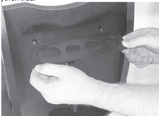
Рисунок 15. Используя два шурупа из комплекта, установите алюминиевую раму для окуляра в высверленные на заводе отверстия рядом с верхней частью переднего основания.
