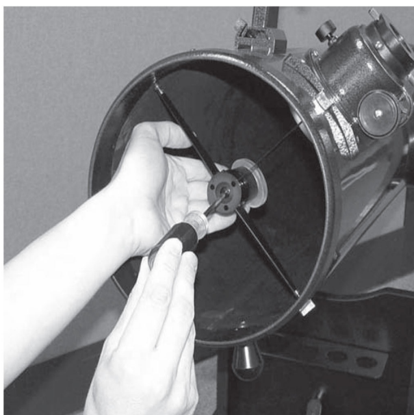
Рисунок 23. Для центрирования вторичного зеркала под фокусировщиком, отрегулируйте центральный винт крестовой отверткой, удерживая пальцами держатель зеркала. Не касайтесь поверхности зеркала
