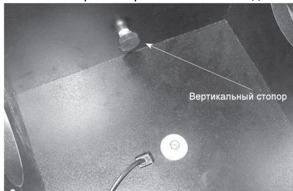
Рисунок 14. Вкрутите вертикальный стопор с шайбами в отверстие с резьбой в передней скобе.
