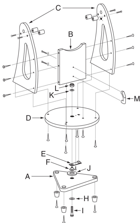
Рисунок 9. Монтировка Добсона в разобранном виде.
