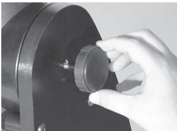
Рисунок 18. Удерживающая ручка с нейлоновой прокладкой вкручивается со стороны основания, на которой нет порта IntelliScope
