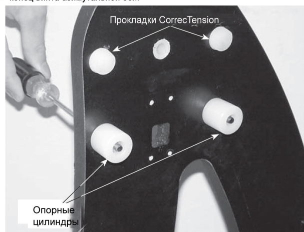
Рисунок 12. Присоединение опорных цилиндров.
