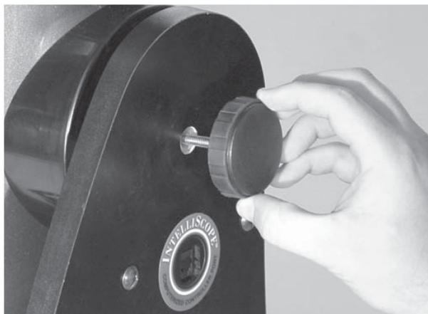
Рисунок 17. Ручка регулировки натяжения с металлической и нейлоновой шайбами, вкручивается со стороны основания, на которой находится порт IntelliScope. Ручку регулировки натяжения следует затягивать до тех пор, пока прокладки CorrectTension не коснутся высотных подшипников телескопа.
