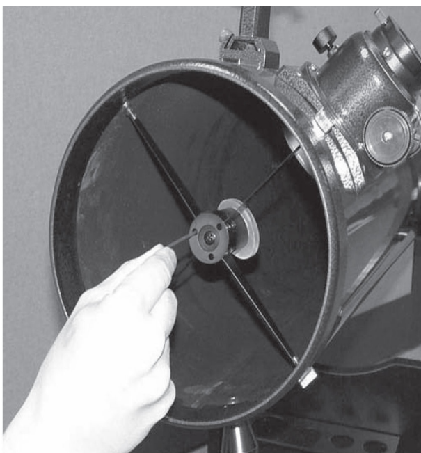
Рисунок 24. Отрегулируйте наклон вторичного зеркала, ослабляя или затягивая регулировочные винты 2 мм шестигранником.
