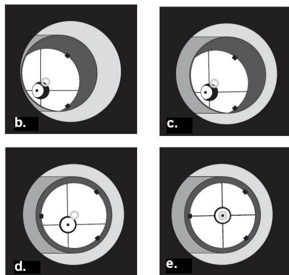
Рисунок 8. Коллимация оптики. (a) Если зеркала выровнены надлежащим образом, Вы должны увидеть похожую картинку. (b) С установленной коллимационной крышкой, если оптика не выровнена, изображение будет выглядеть так. (c) Здесь, вторичное зеркало центрировано, но требуется отрегулировать его наклон, чтобы видеть отражение основного зеркала. (d) Вторичное зеркало окончательно выровнено, но основное зеркало нуждается в регулировке. Когда оно будет выровнено, "точка" будет находиться точно в центре (e).
