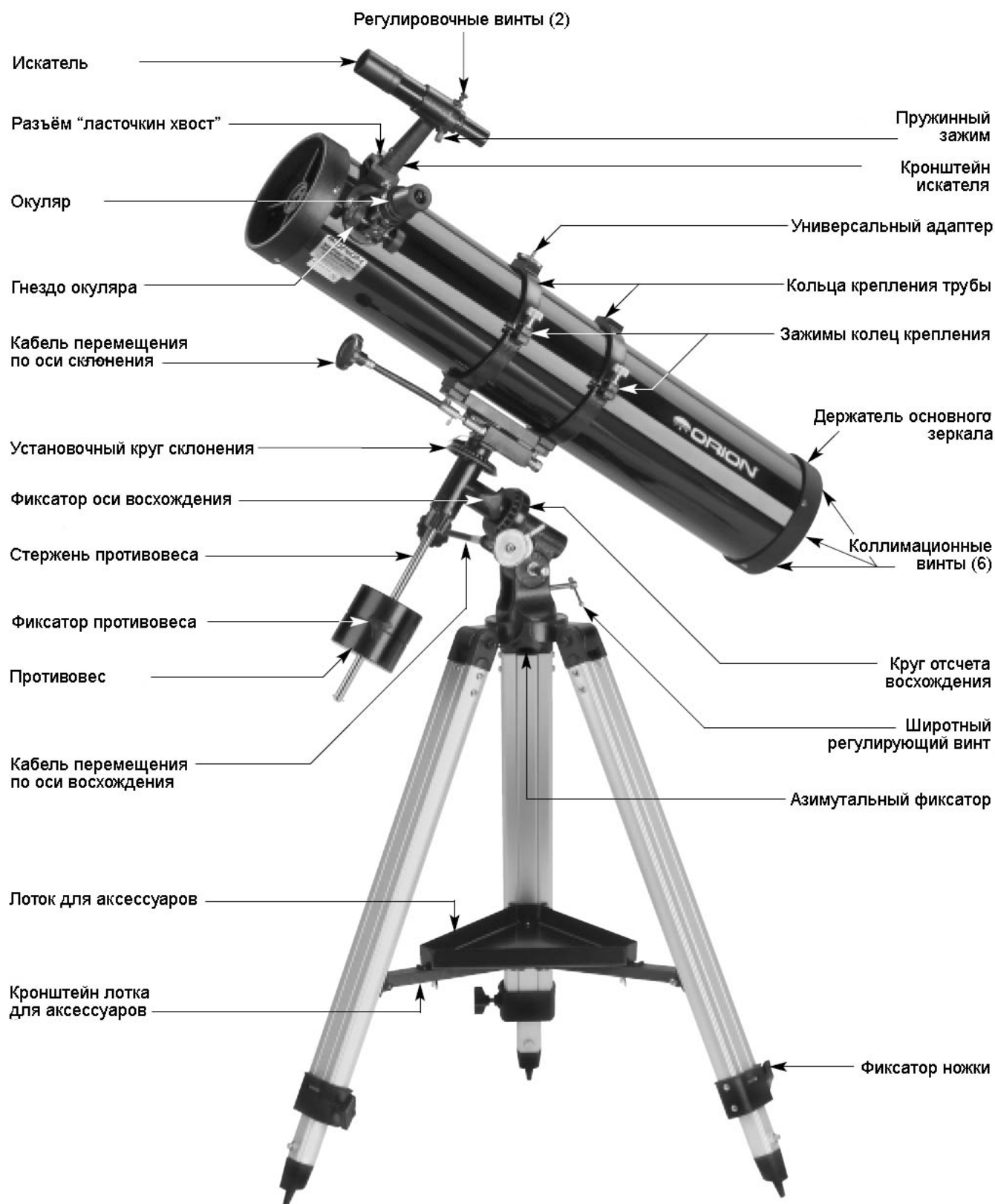
Рисунок 1. SpaceProbe 130 EQ
