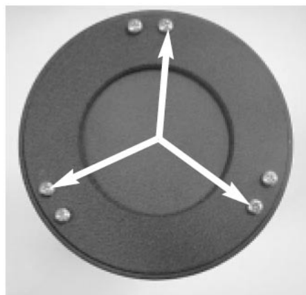
Рисунок 15. Выньте три коллимационных винта, отмеченных стрелками, для снятия зеркала.
