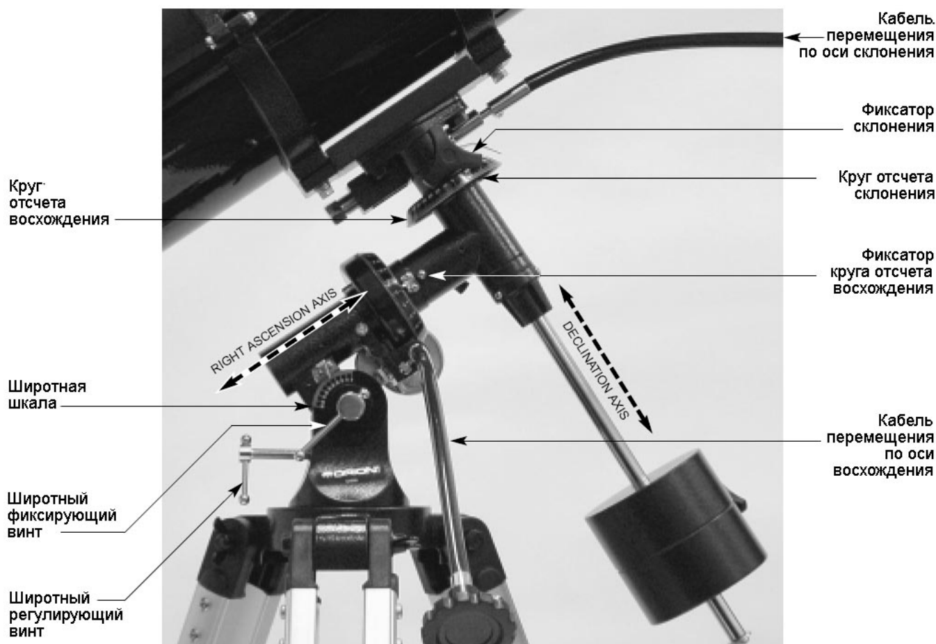
Рисунок 2. экваториальное крепление SpaceProbe 130
