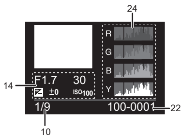
Отображение гистограммы
