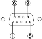
Внешний вид 9-контактного разъема D-SUB
