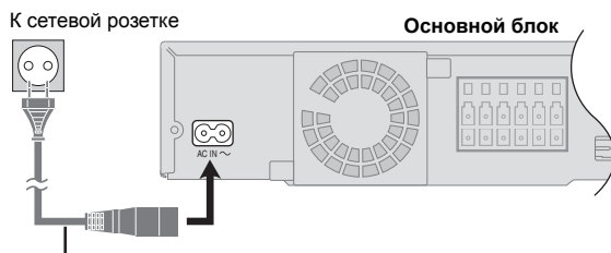
Сетевой шнур (входит в комплект поставки)
