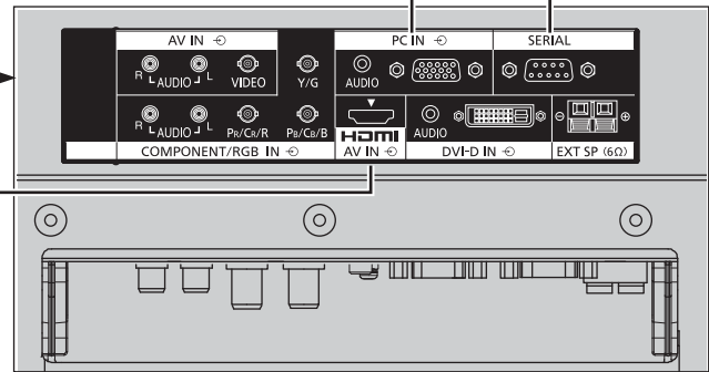
Разъемы в нижней части плазменного дисплея.
