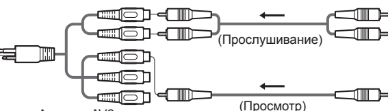
Адаптер AV2 (COMPONENT / VIDEO) (входит в комплект поставки)
