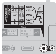
Адаптер AV2 (COMPONENT / VIDEO) (входит в комплект поставки)
