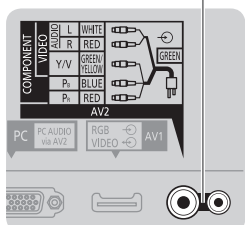
Задняя панель телевизора
