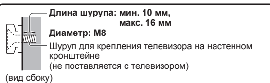
Отверстия для крепления настенного кронштейна
