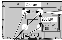
Отверстия для крепления настенного кронштейна
