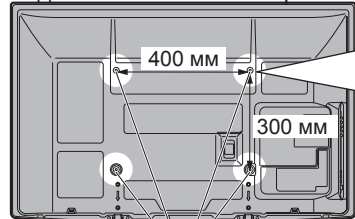
Задняя панель телевизора
