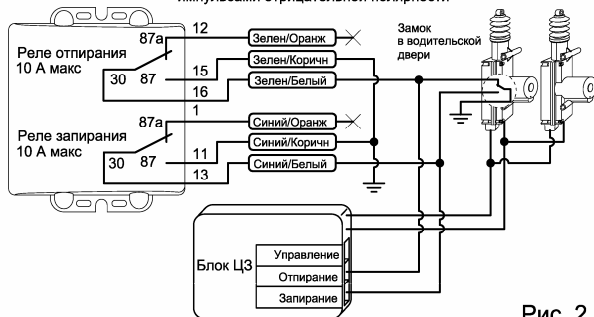
Схема подключения в автомобилях с пневмоэлектрическим компрессором центрального замка : AUDI, MERCEDES
