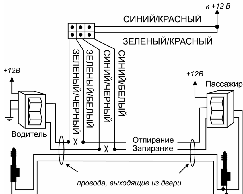
Схема 3. 5 (4) проводная система с обратной (переменной) полярностью (большинство легковых а/м марки Форд и Крайслер; большинство грузовых а/м марки Форд и GM)
