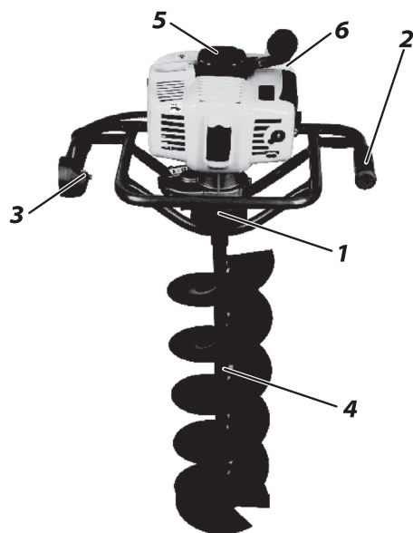
Модели AE 51D / AE 53D / AE 70D
