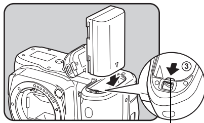
Защелка аккумулятора
